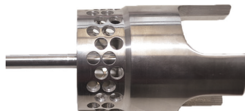
bælz 340-2-B cage plug
