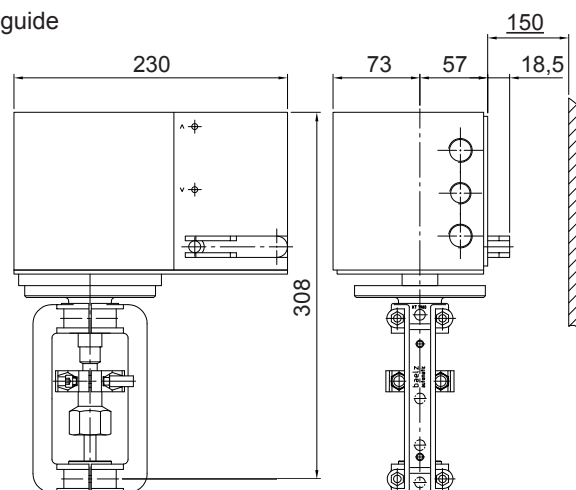
Dimensions of bælz 373-E65 actuator
