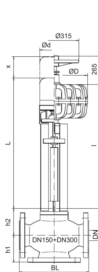
bælz 347-BBK DN150-300 bælz 347-BBK-SS DN150-300
